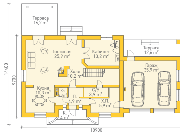
Экспликация | 1 этаж
