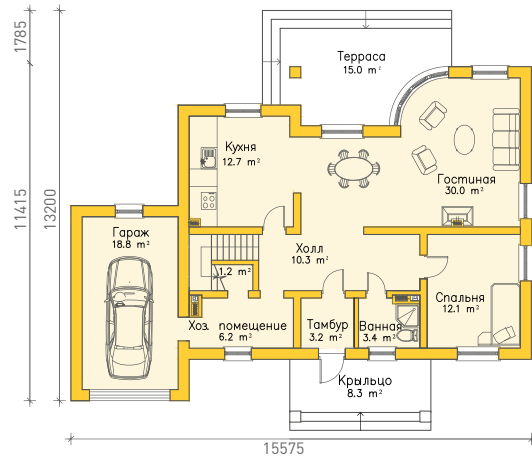
Экспликация | 1 этаж
