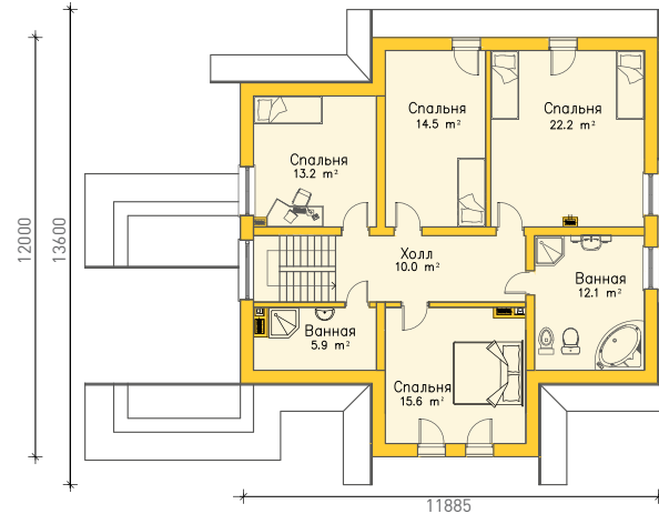
Экспликация | 2 этаж
