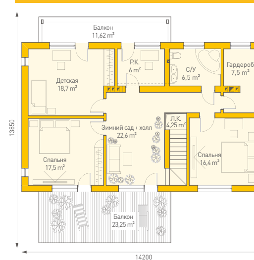
План | 2 этаж
